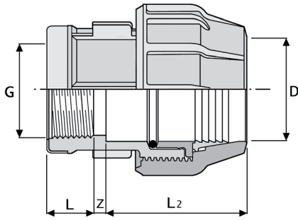
601 Raccordo femmina
