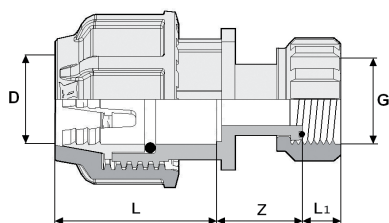
525 Adattatore a ghiera
