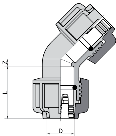
526 Gomito a 45°
