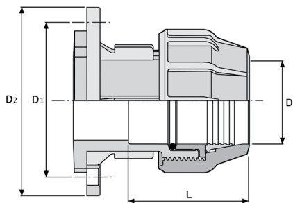
520 Giunto flangiato
