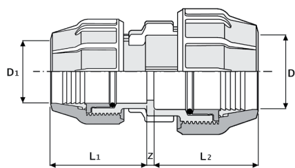
512 Manicotto ridotto
