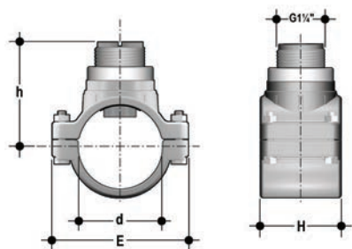
SVLC Prese a staffa serie BS
