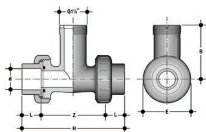
TFAV Raccordi a T in PVC serie ASTM SCH. 80 (attacchi femmina per incollaggio - PN10)
